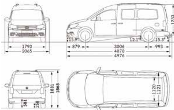
尺寸圖
