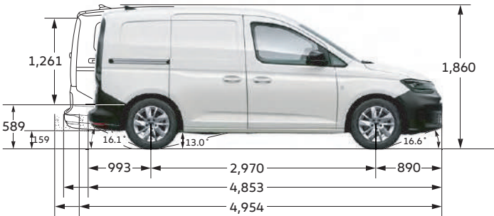
Caddy Cargo 長軸尺寸圖 (此圖圖式為示意)
