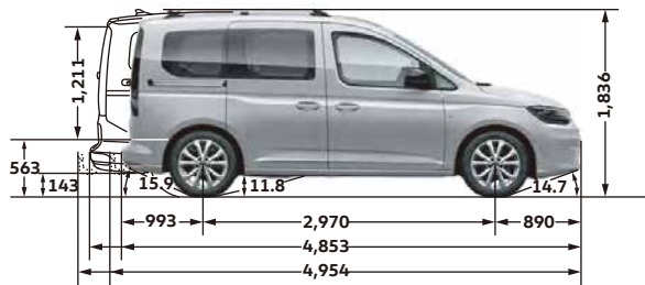
Caddy Maxi 尺寸圖
