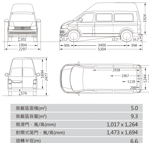
Kombi長軸高頂尺寸圖
