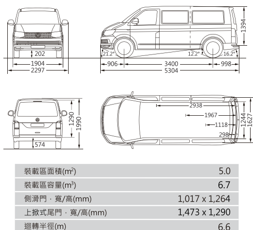
Kombi長軸平頂尺寸圖
