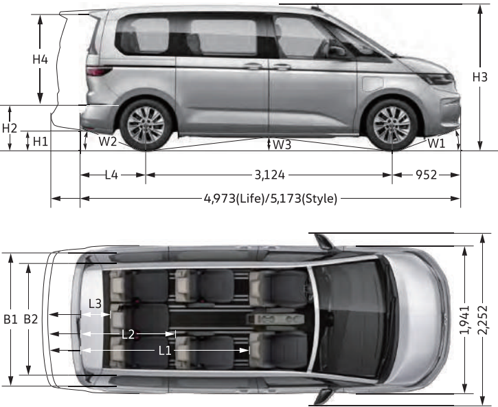
New Multivan 尺寸圖
