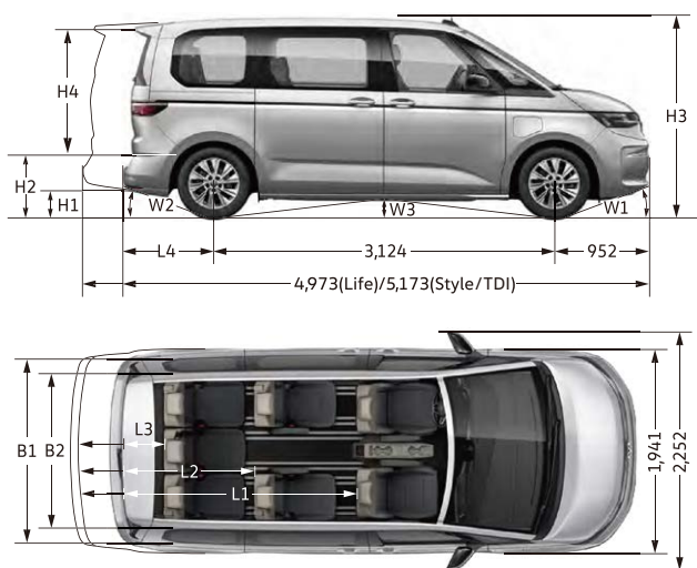
New Multivan 尺寸圖
