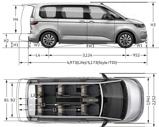
New Multivan 尺寸圖
