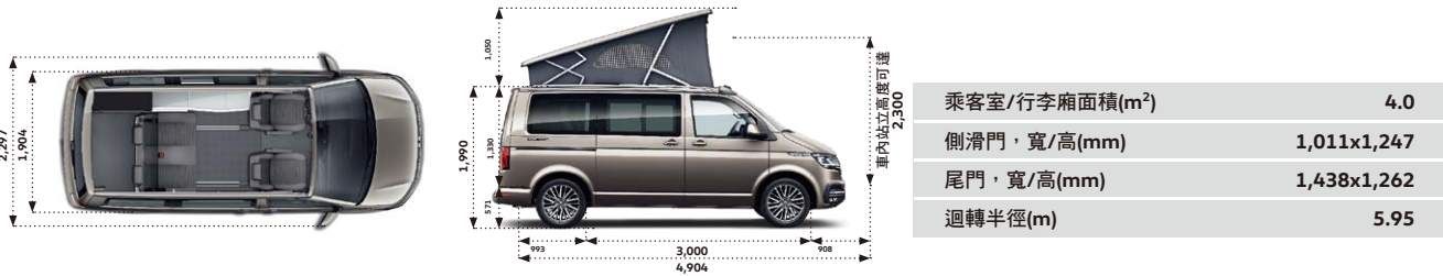
T6.1 California Ocean 4MOTION 尺寸圖
