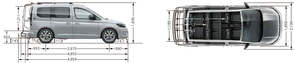
Caddy Maxi 尺寸圖
