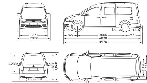
Caddy Maxi 尺寸圖
