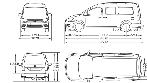
Caddy Maxi 4MOTION 尺寸圖
