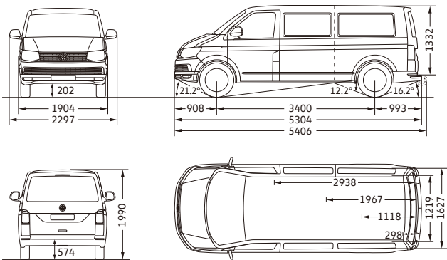
Caravelle L (長軸版) 尺寸圖
