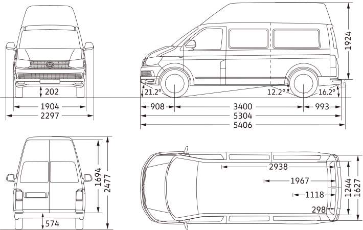
Kombi尺寸圖
