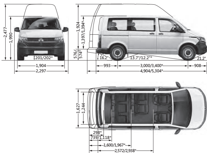
Kombi 尺寸圖
