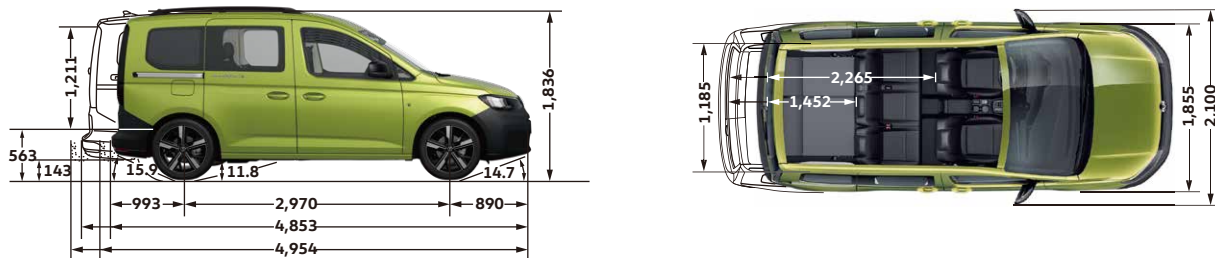
Caddy California 尺寸圖 (單位：mm)
